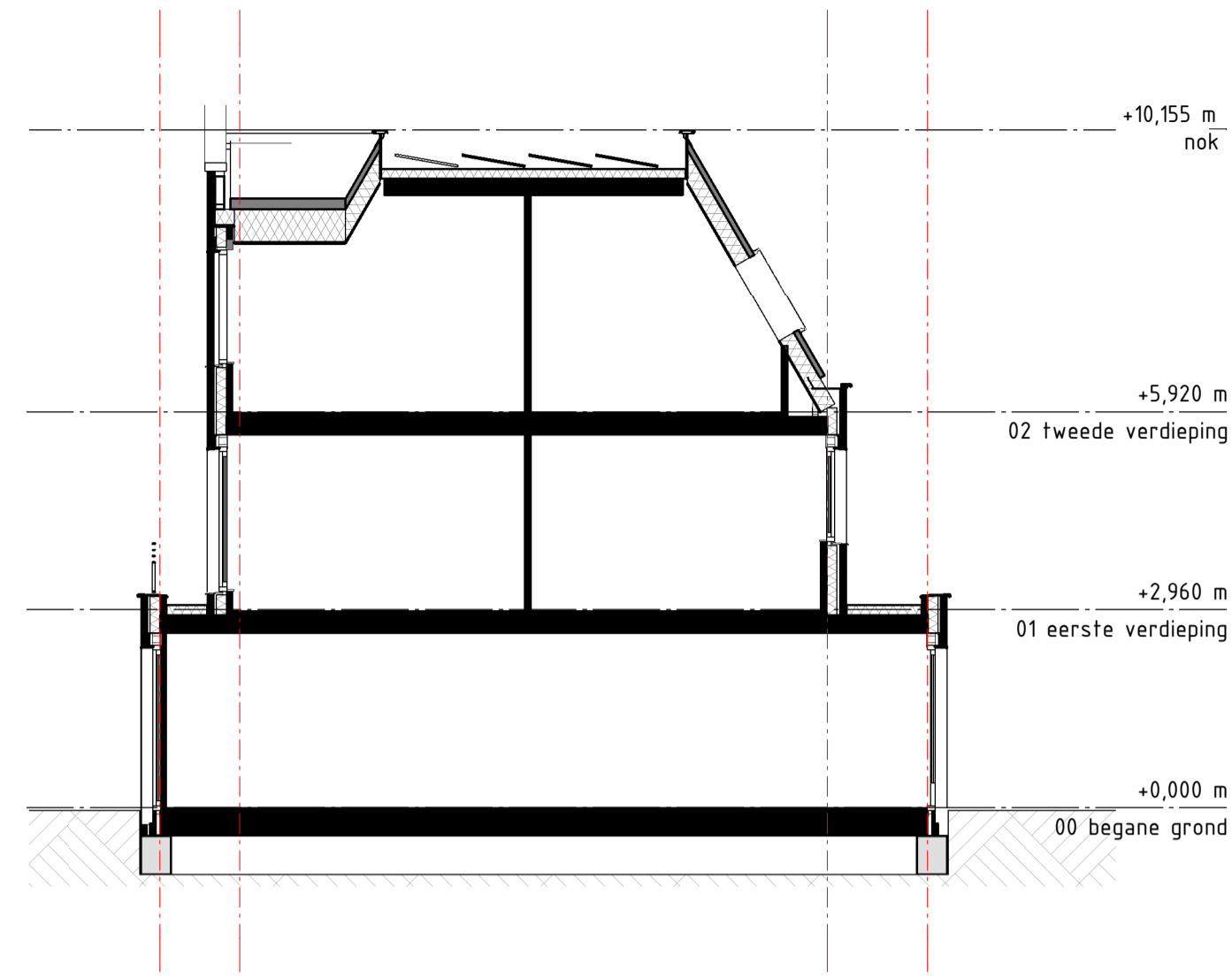
DOORSNEDE 1:100 TYPE C1'
