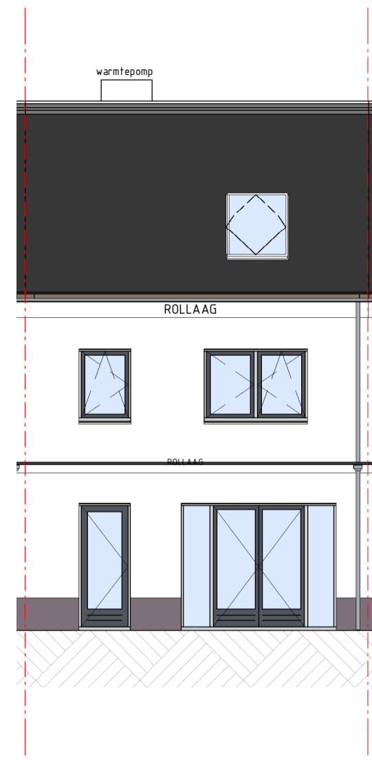
ACHTERGEVEL 1:100 TYPE C1'
