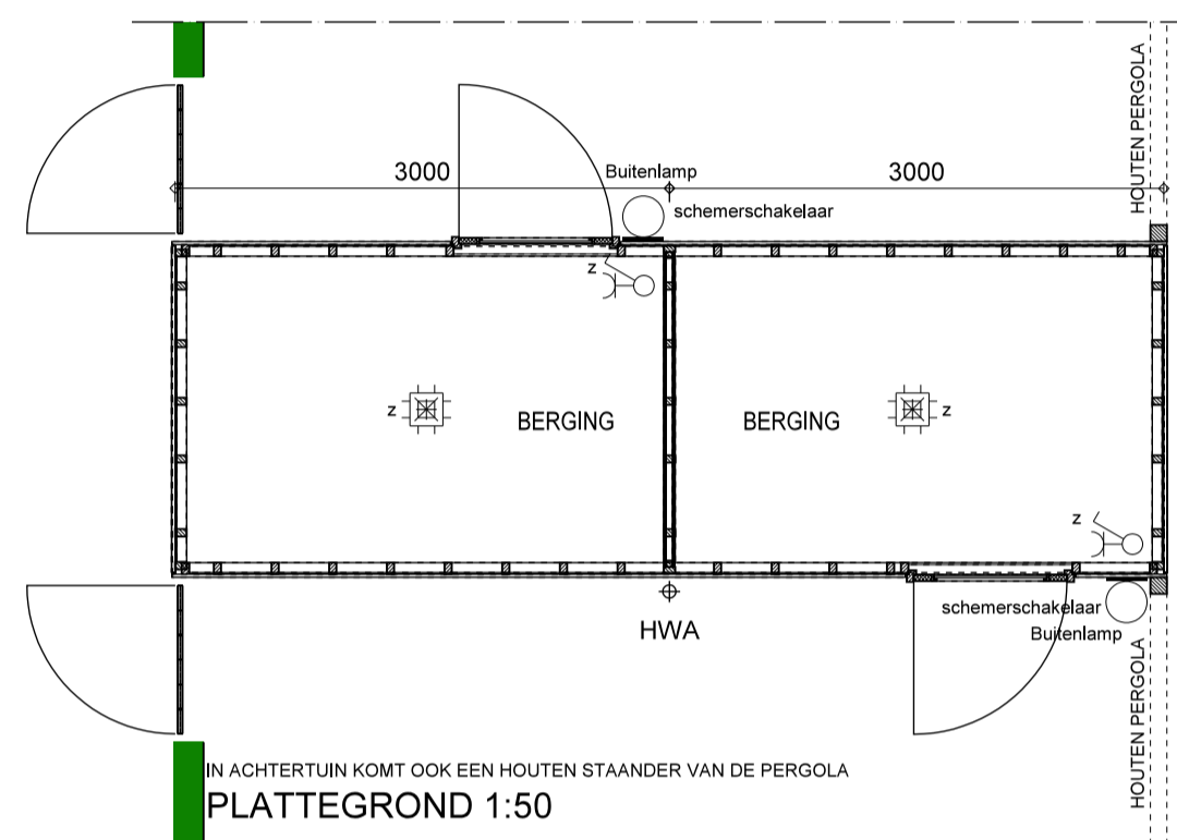
PLATTEGROND 1:50
