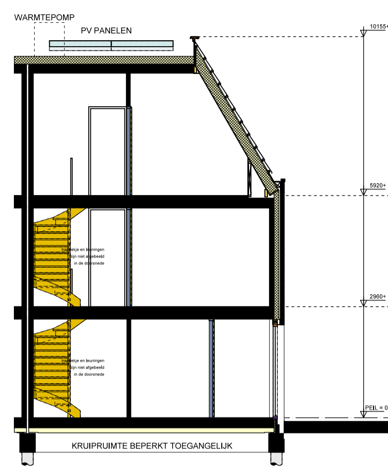
DOORSNEDE 1:100
