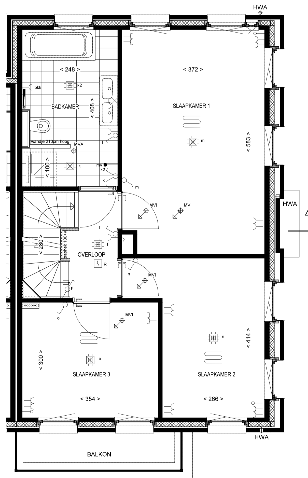
PLATTEGROND 1:50
