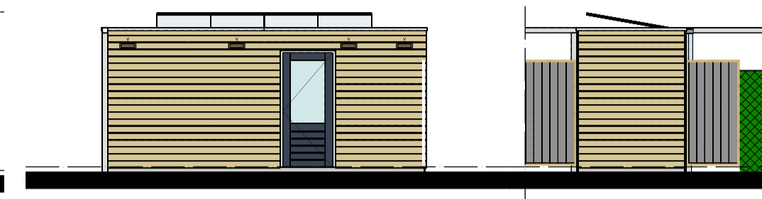
ACHTERGEVEL 1:100
